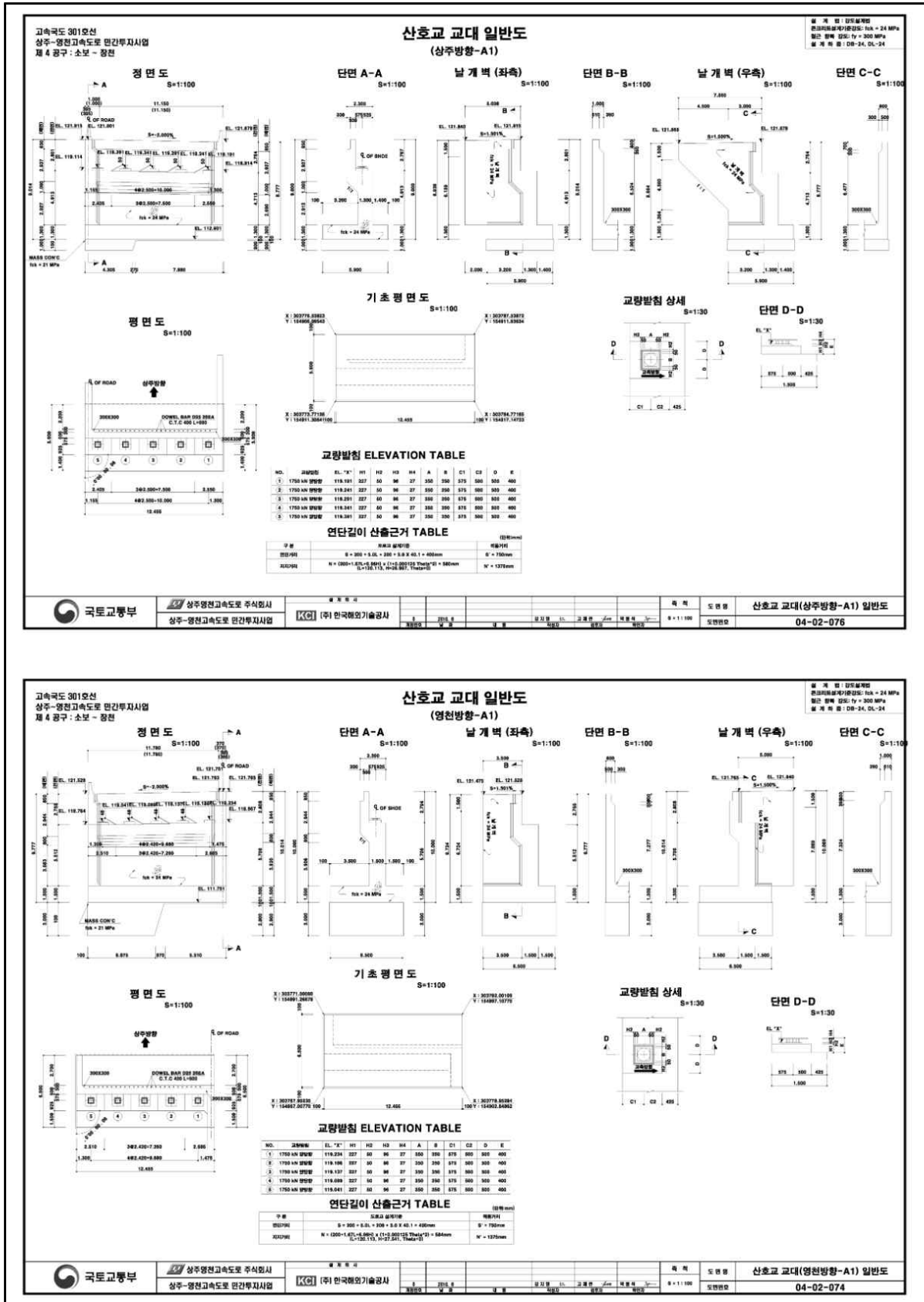
【그림 8.1.6】 교대 일반도
